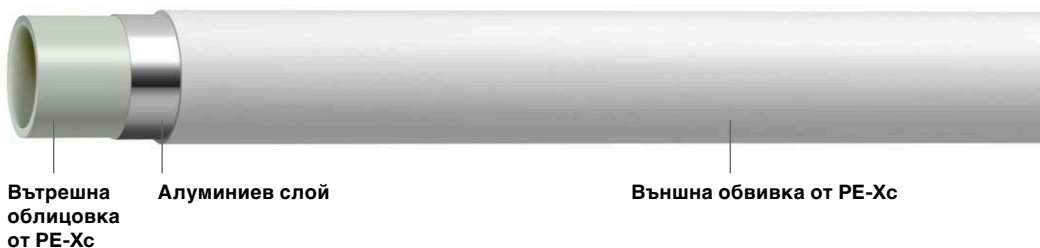
Конструкция на тръбата Viega Smartpress.
